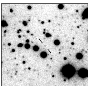
MRC B0647-475
