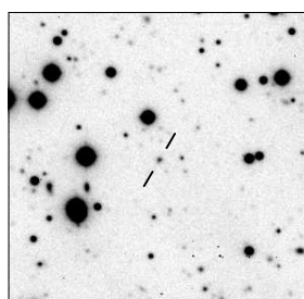
MRC B0700-473
