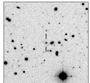
MRC B0420-625
