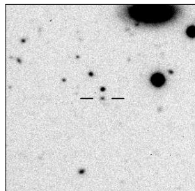
MRC B0411-346A
