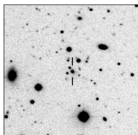
MRC B0601-344
