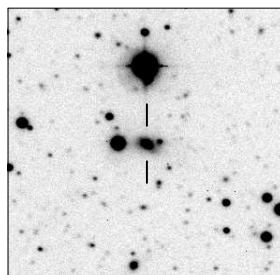
MRC B0436-650
