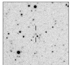
MRC B0546-445
