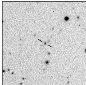
MRC B0335-415
