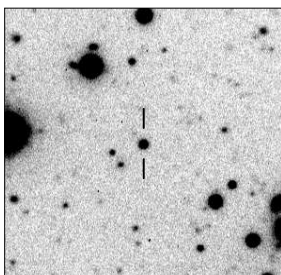
MRC B0427-366
