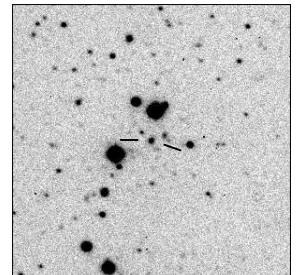
MRC B0407-658
