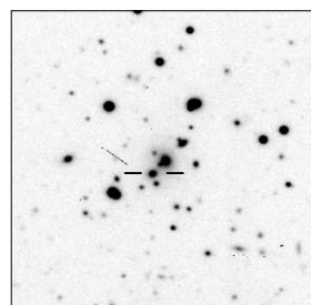
MRC B0614-349
