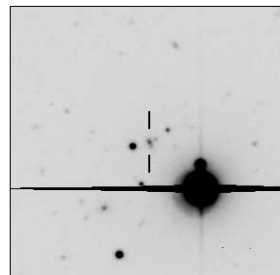
MRC B0411-561
