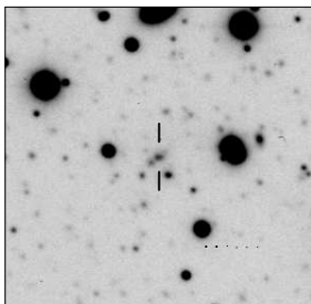
MRC B0409-752
