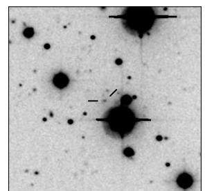
MRC B0615-365
