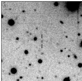
MRC B0315-685
