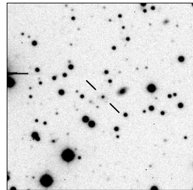
MRC B1017-421
