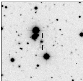
MRC B1030-340
