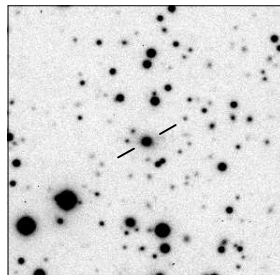
MRC B1143-483
