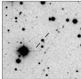
MRC B1015-314
