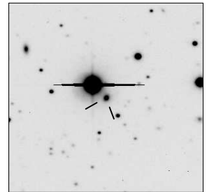
MRC B1017-325
