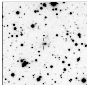
MRC B1526-423
