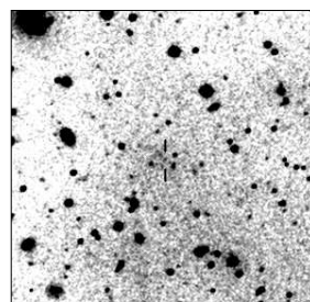
MRC B1721-836
