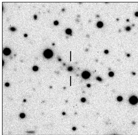
MRC B1359-358
