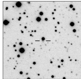
MRC B1445-468
