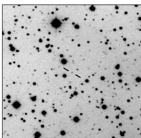
MRC B1706-606
