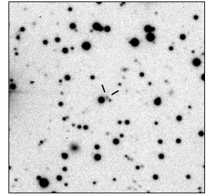
MRC B1358-493
