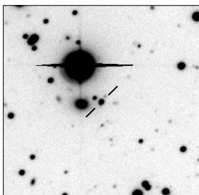
MRC B1547-795
