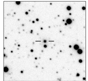
MRC B1451-364
