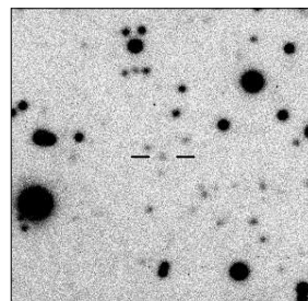
MRC B1607-841
