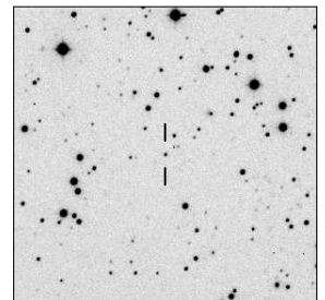
MRC B1540-730
