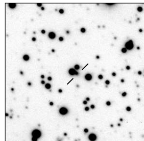
MRC B1540-337
