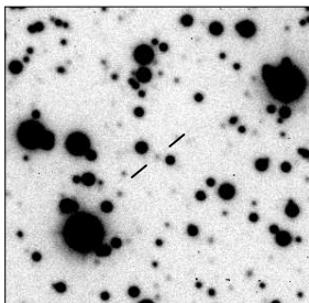
MRC B1458-391
