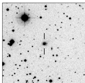
MRC B1716-800
