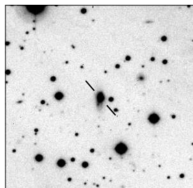
MRC B1549-790
