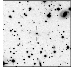
MRC B1818-557
