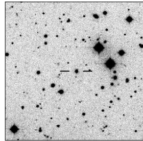
MRC B1854-663
