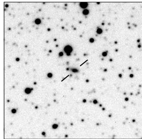
MRC B1827-360
