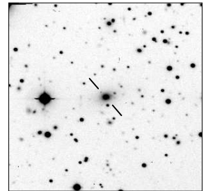
MRC B1831-668
