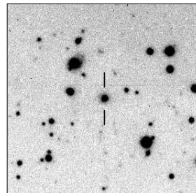
MRC B1932-464
