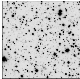
MRC B1853-303
