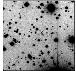
MRC B1756-663
