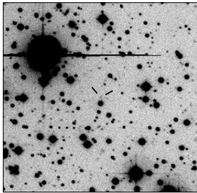
MRC B1840-404
