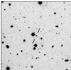
MRC B1922-627
