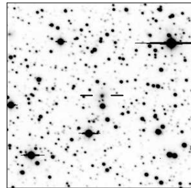
MRC B1829-344
