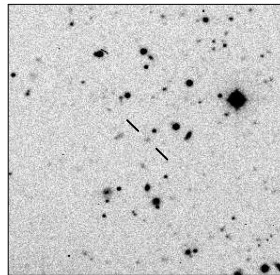
MRC B2059-641
