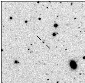
MRC B2041-604
