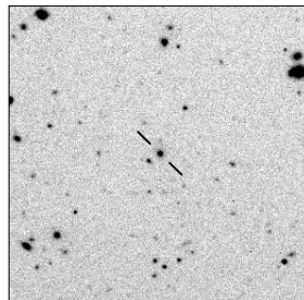
MRC B2305-418
