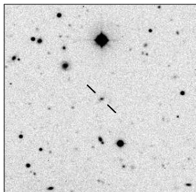
MRC B2150-520
