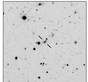
MRC B2032-350
