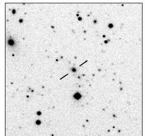
MRC B2201-555
