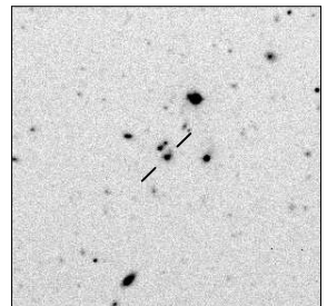
MRC B2252-530
