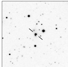
MRC B2020-575
