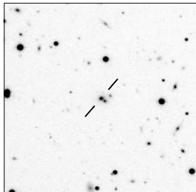
MRC B2009-524
