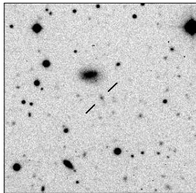
MRC B2049-368
