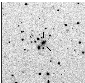
MRC B2223-528
