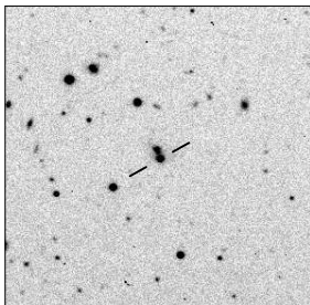
MRC B2253-522
