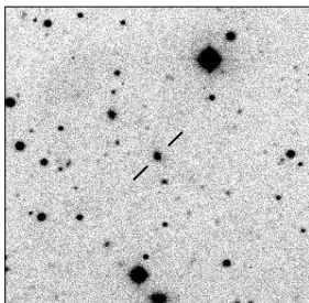
MRC B2140-817
