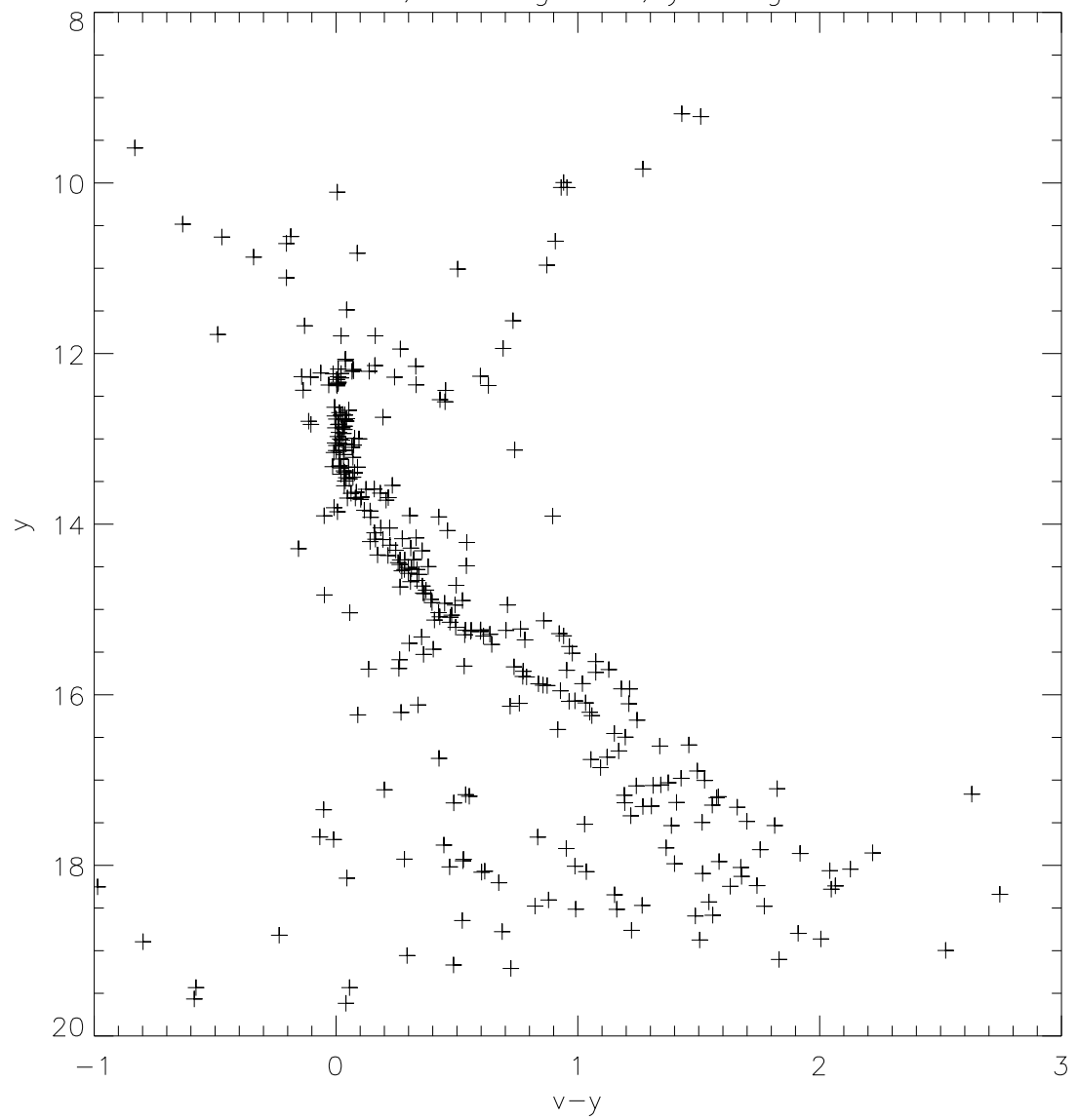
M67, Stromgren v, y images
